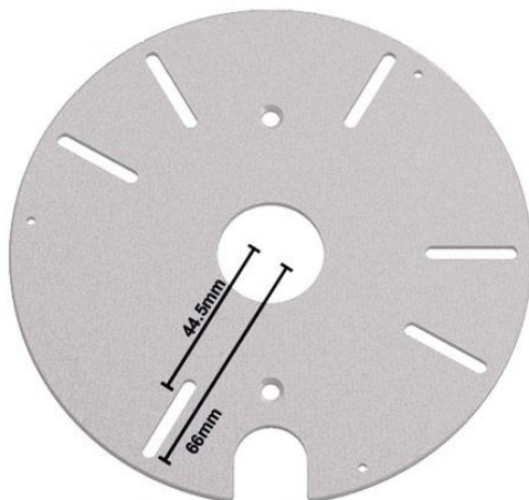
Montageplatte für Bohrlocher-Radius 44.5 - 66mm
