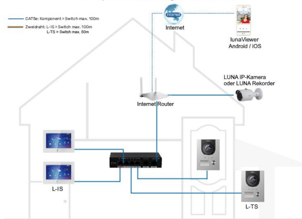
Beispiel Verkabelung IP-Netzwerk
